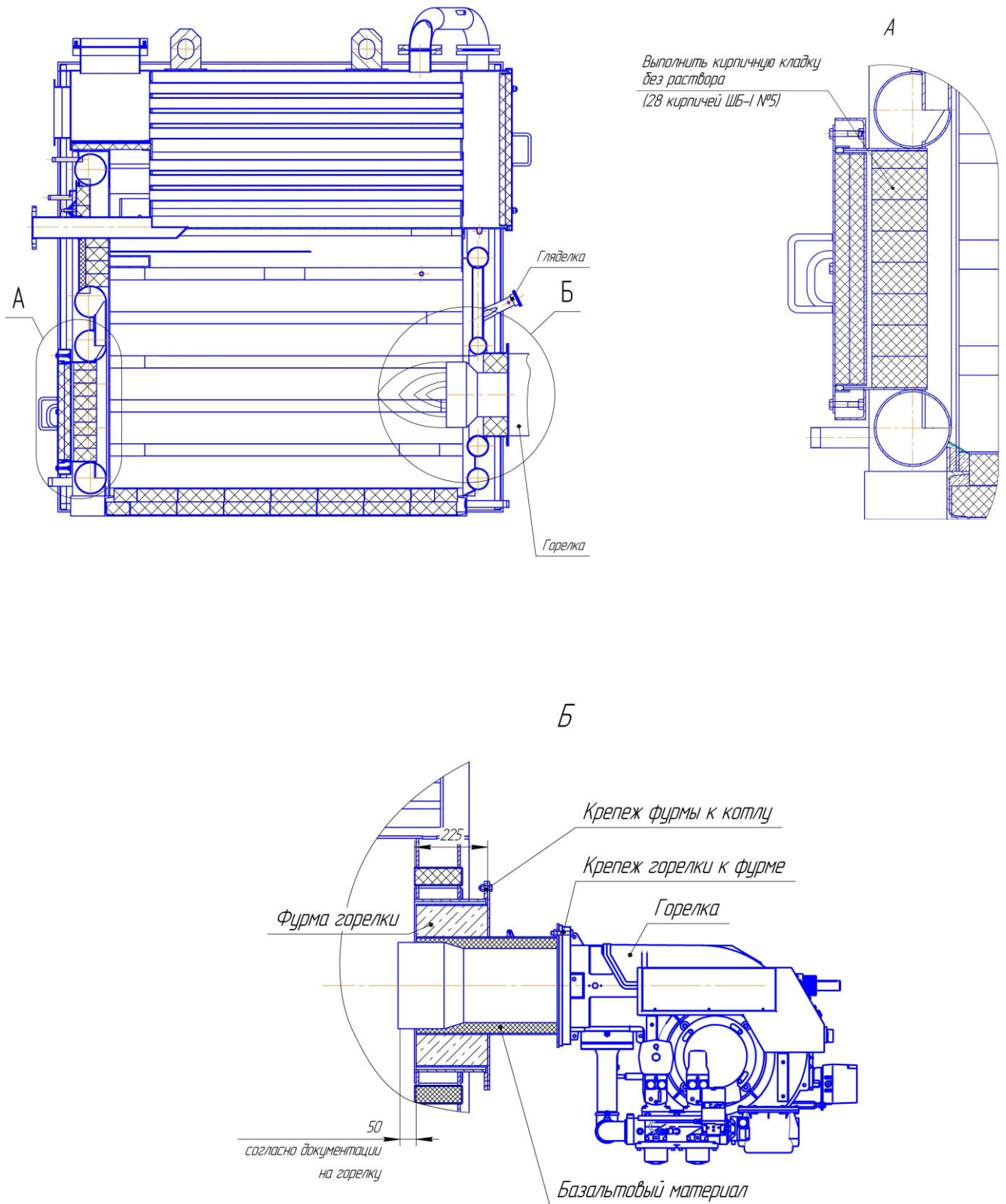
Рис. 2 Огнеупорная защита из кирпича и установка горелки
