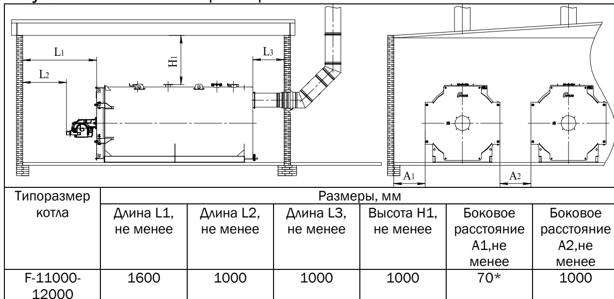
Рисунок 7. Установочные размеры
