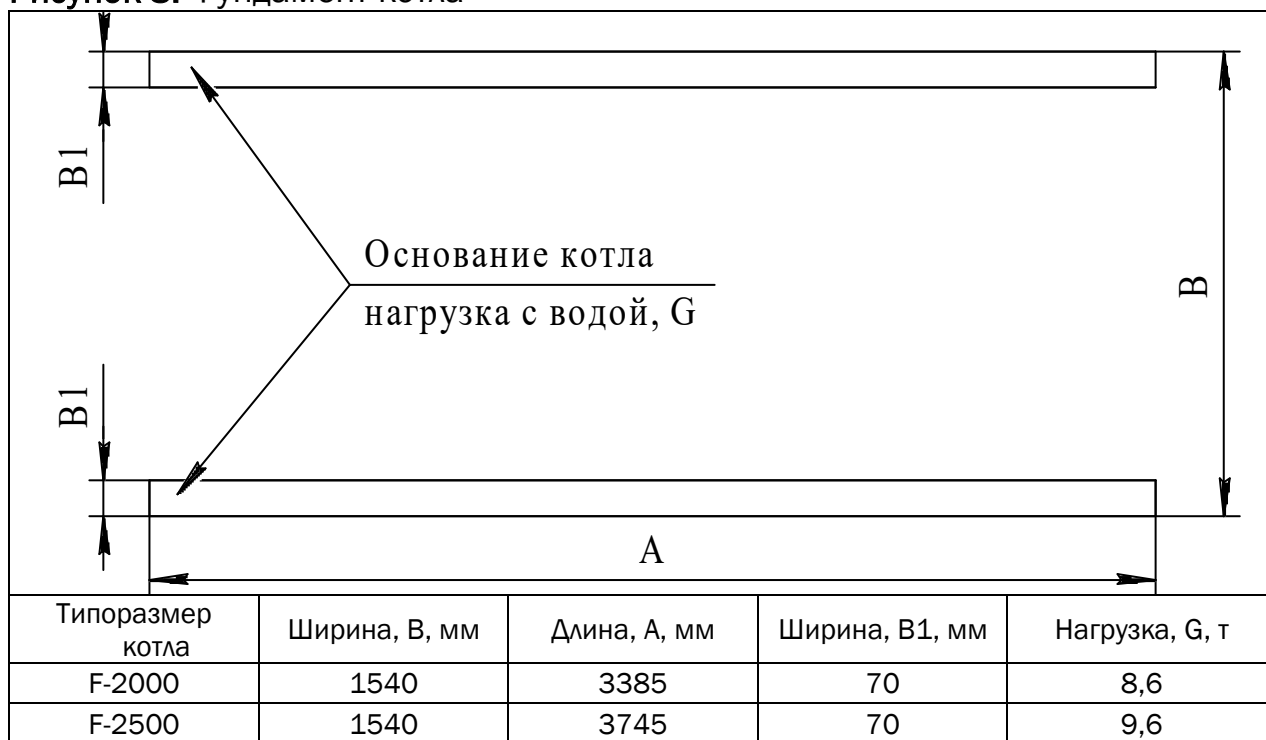
Рисунок 8. Фундамент котла
