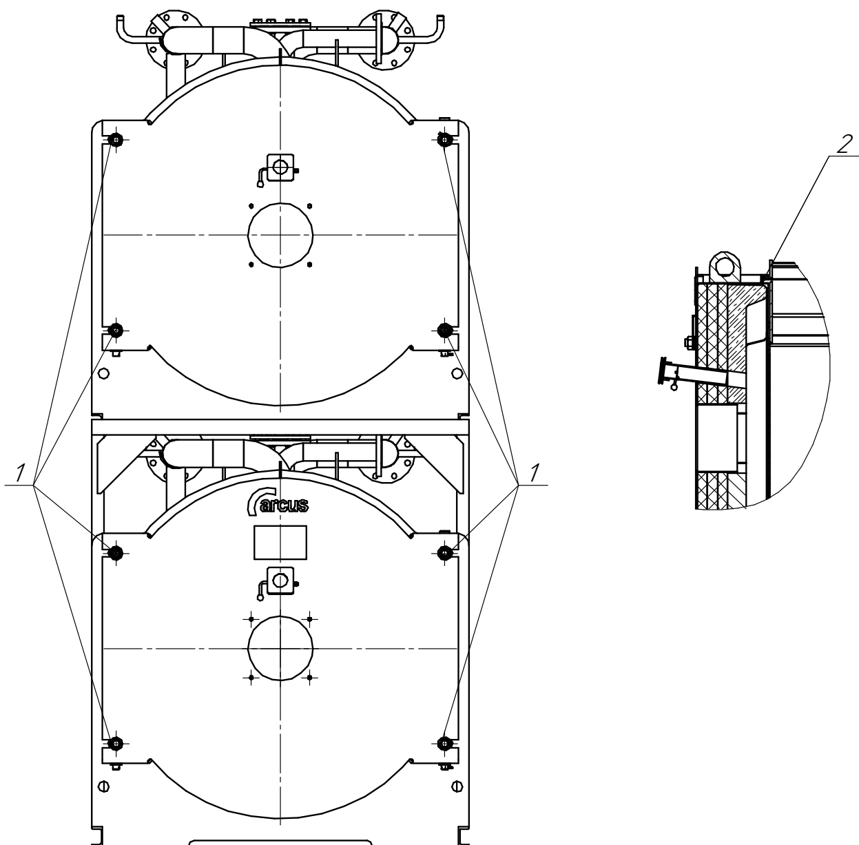
Рисунок 10. Передние крышки.
