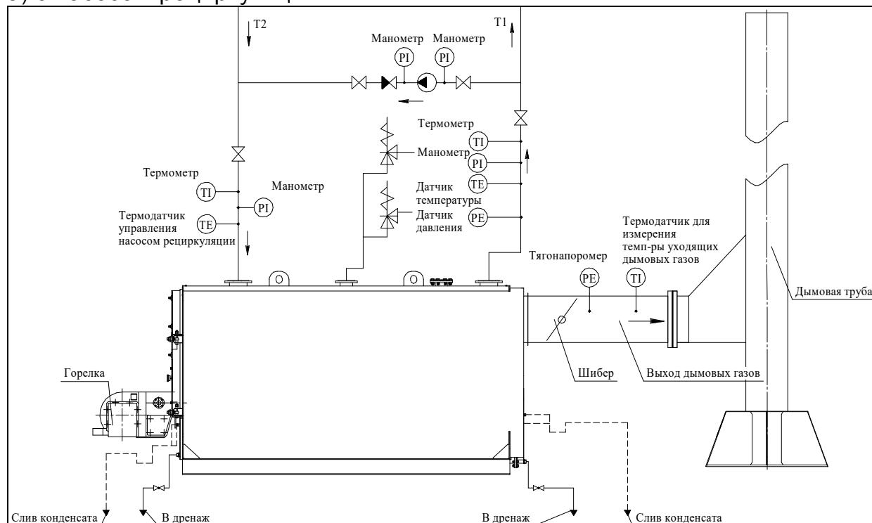
Рисунок 6. Принципиальные схемы включения котла:
