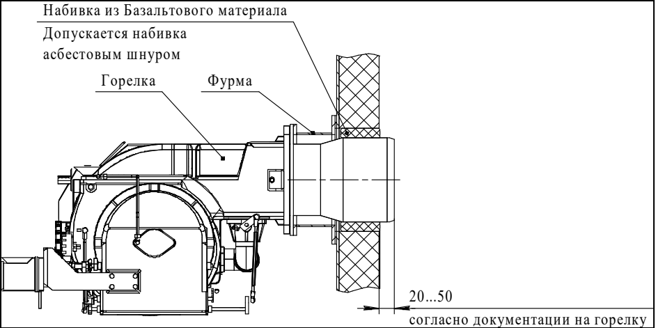
Рисунок 3. Крепление горелки
