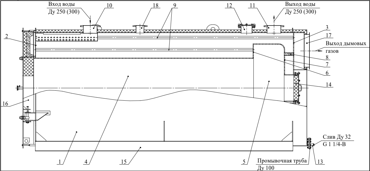
Рисунок 1. Схема котла
