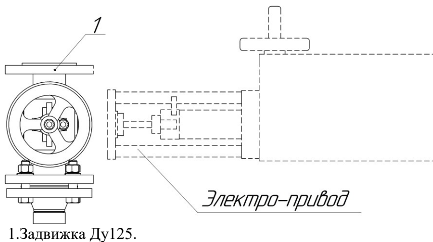
Рис. 10. Выход пара
