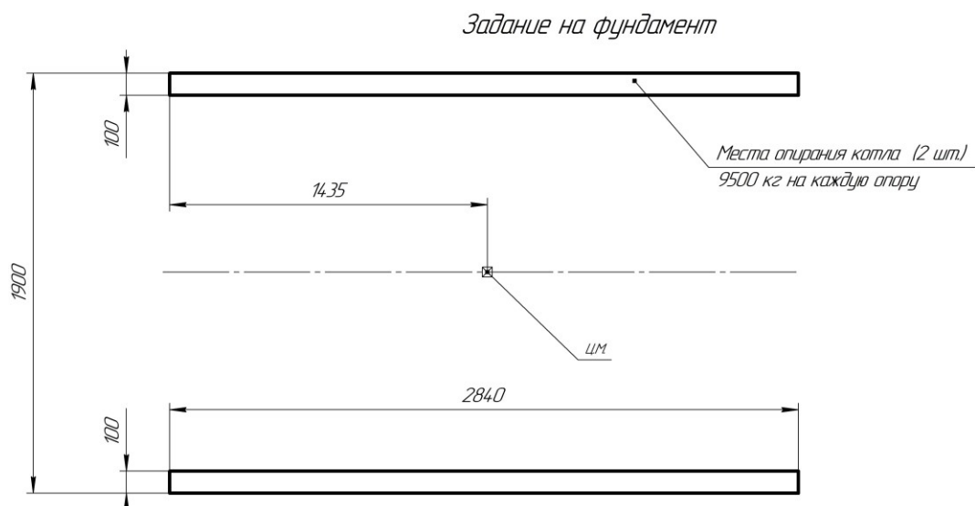
Рисунок 19. Опорные места котла.
