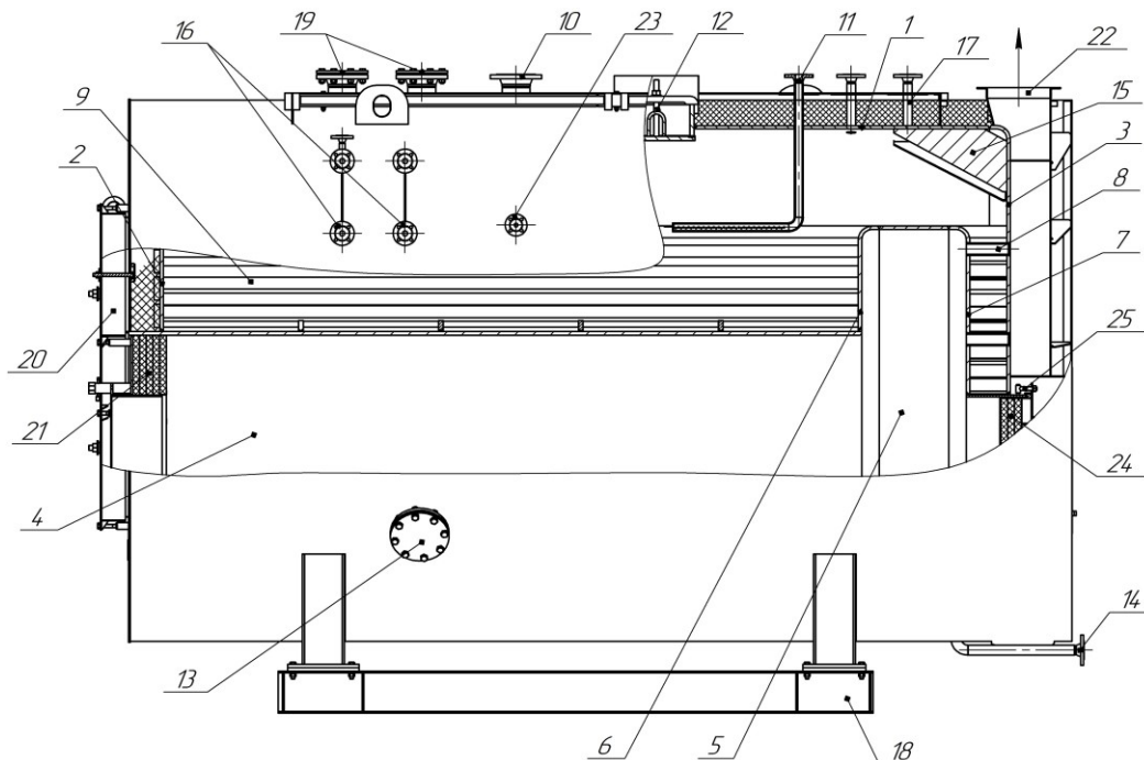
Рис. 14. Схема котла
