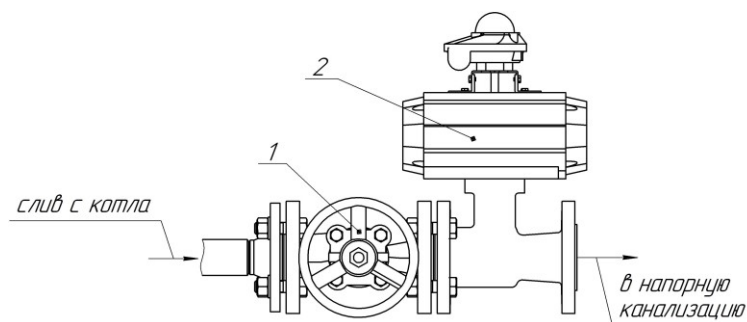
1. Запорный вентиль Ду40, 2. Клапан продувки с пневмоприводом Ду40
