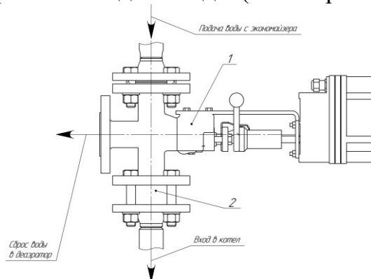
1.Клапан регулирующий подачу воды с электроприводом Ду32, 2. Обратный клапан Ду32.
