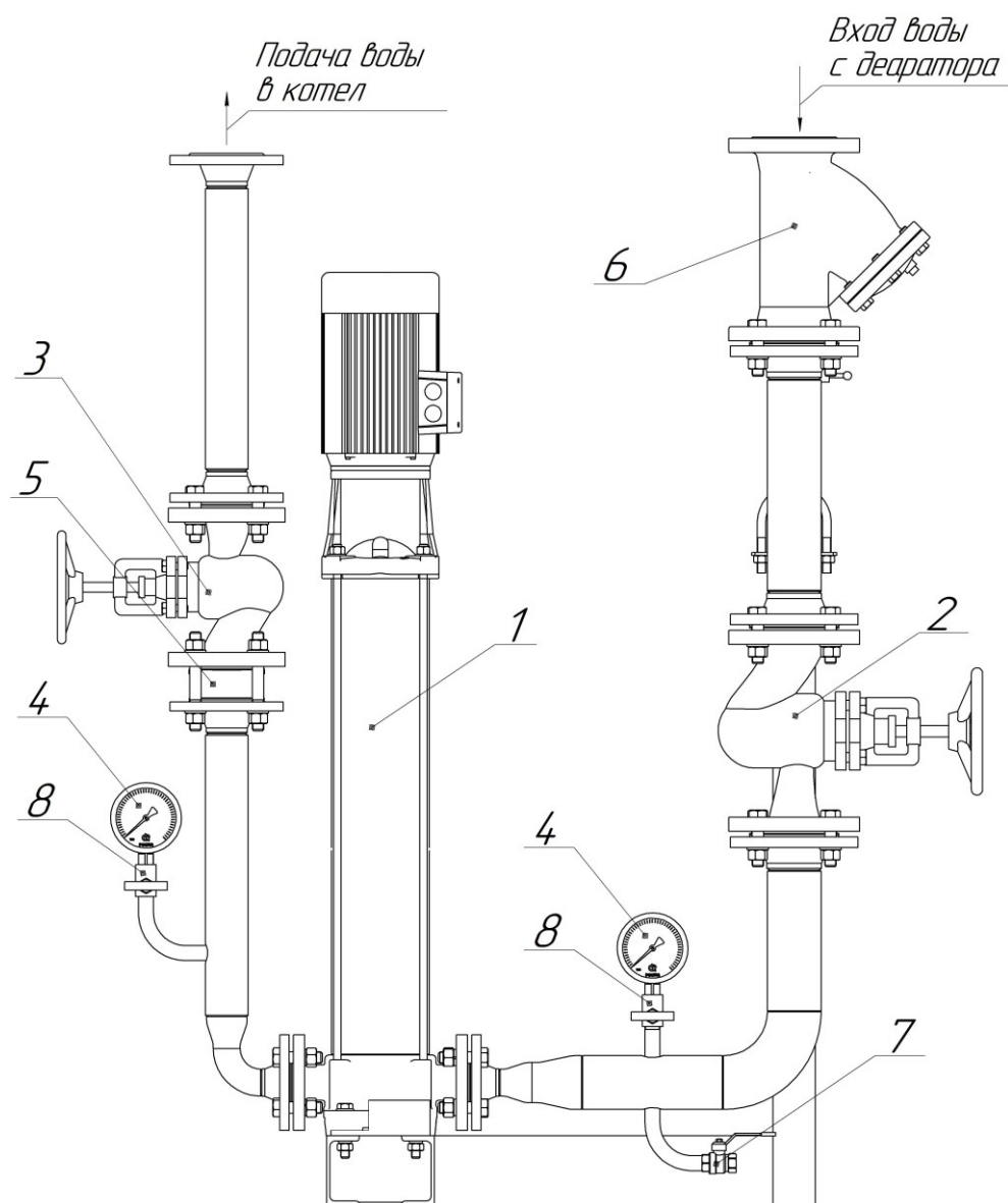
1. Питательный насос, 2. Запорный вентиль Ду65, 3. Запорный вентиль Ду50, 4. Манометр, 5. Обратный клапан Ду50, 6. Фильтр Ду65, 7. Дренажный патрубок Ду15, 8. Игольчатый клапан.
