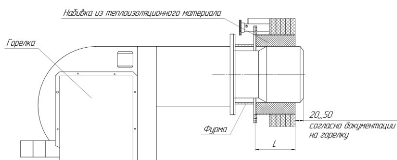
Рис. 16. Крепление горелки
