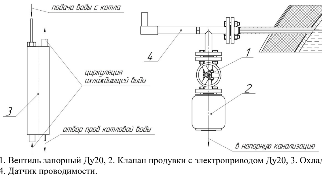
Рис. 11. Непрерывная продувка
