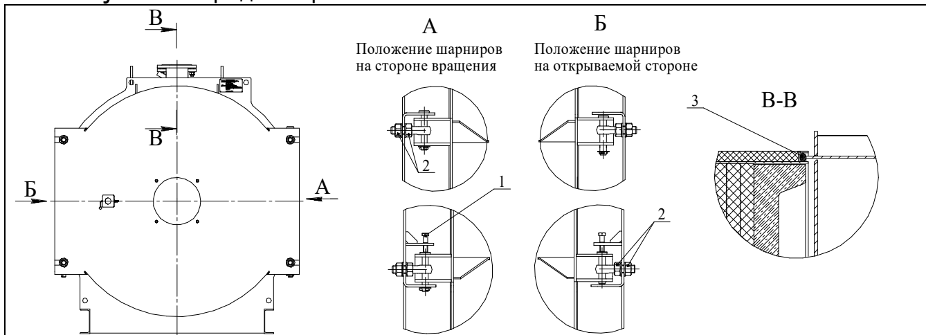
Рисунок 9. Передняя крышка.
