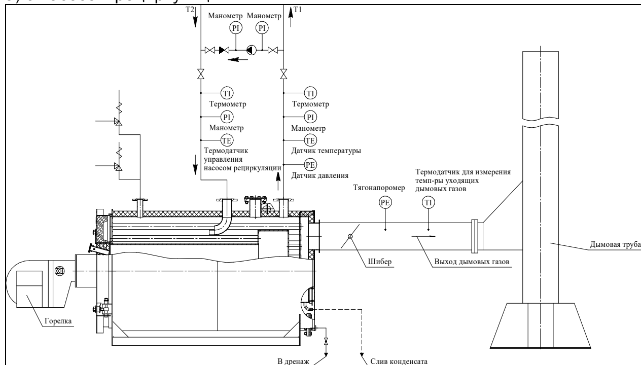
Рисунок 7. Принципиальные схемы включения котла:
