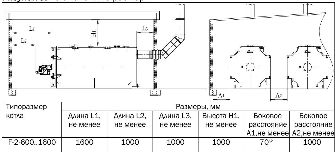
Рисунок 9. Установочные размеры.
