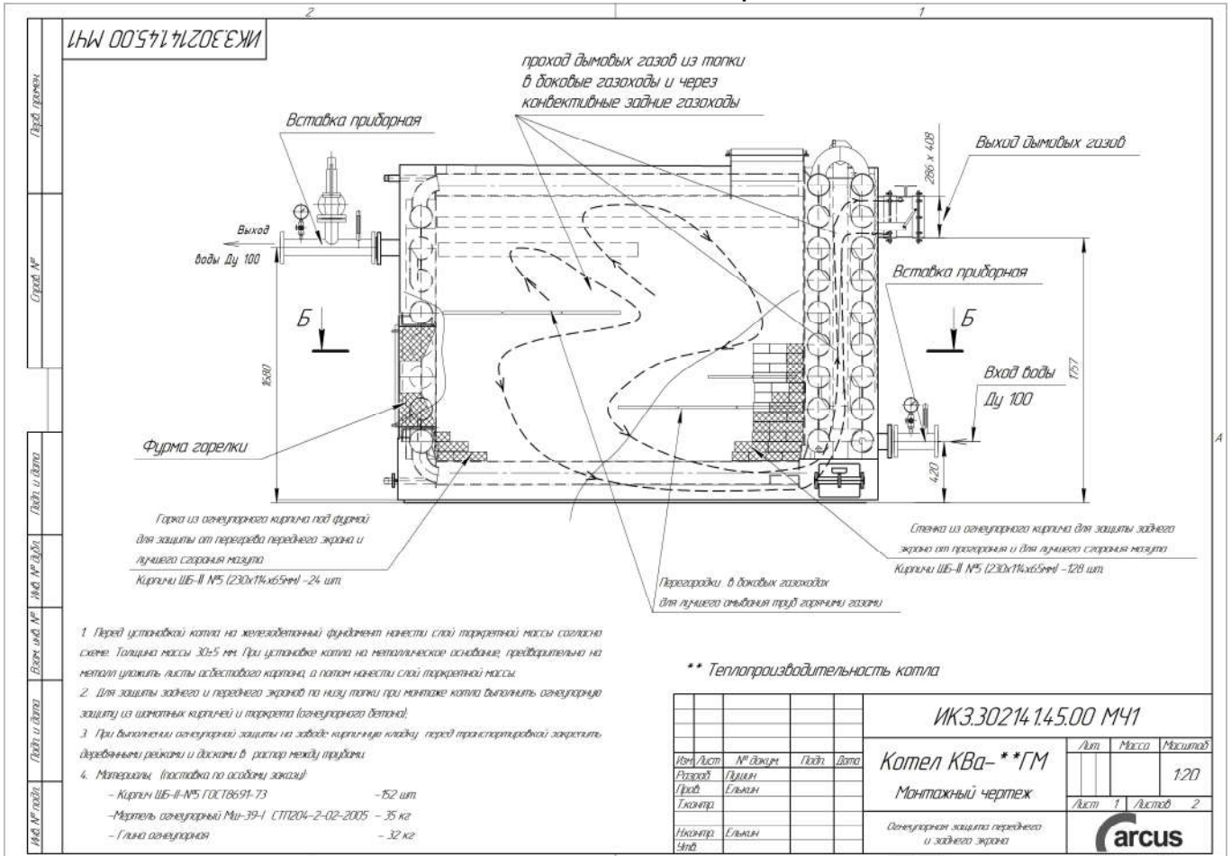
Рис.3 Монтажный чертеж
