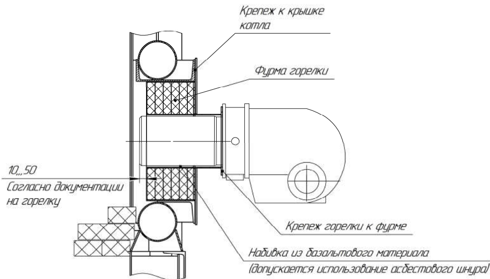
Рисунок 1. Крепление горелки.
