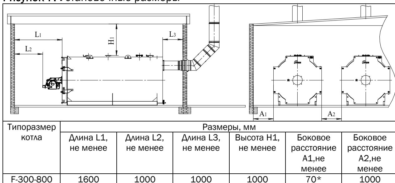
Рисунок 7. Установочные размеры
