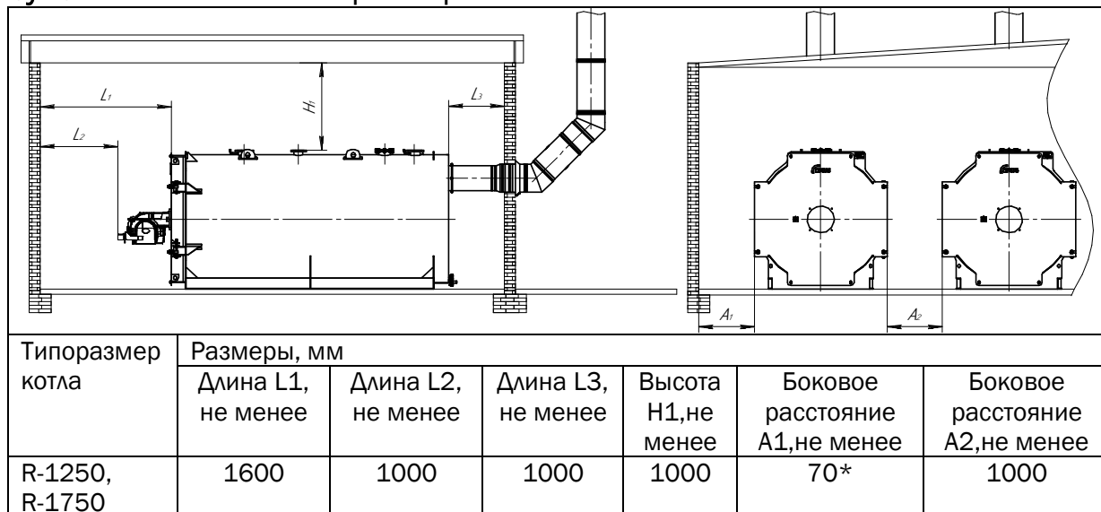
Рисунок 7. Установочные размеры.
