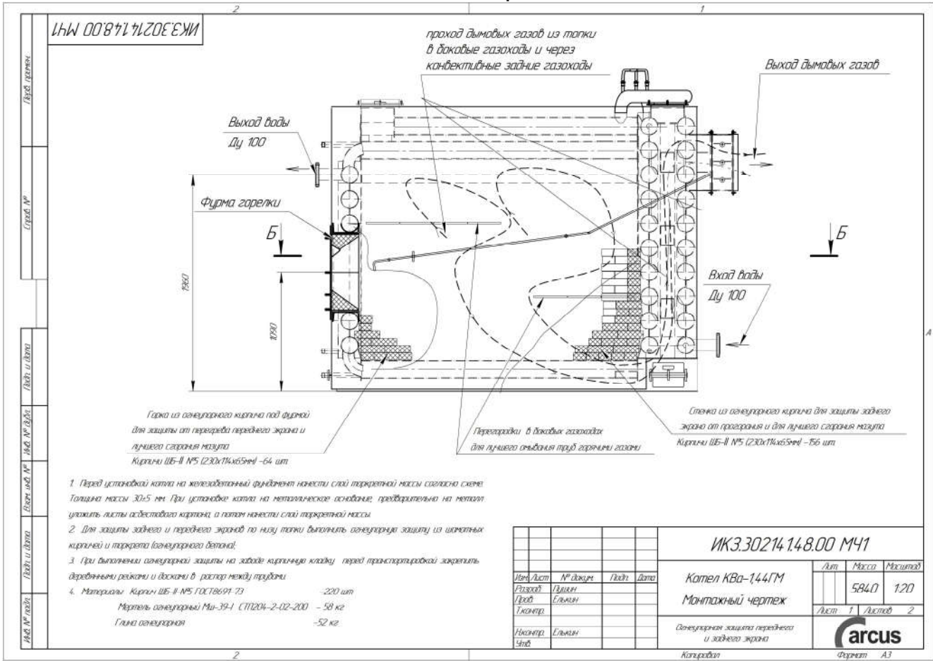
Рис.4 Монтажный чертеж КВа-1,44ГМ
