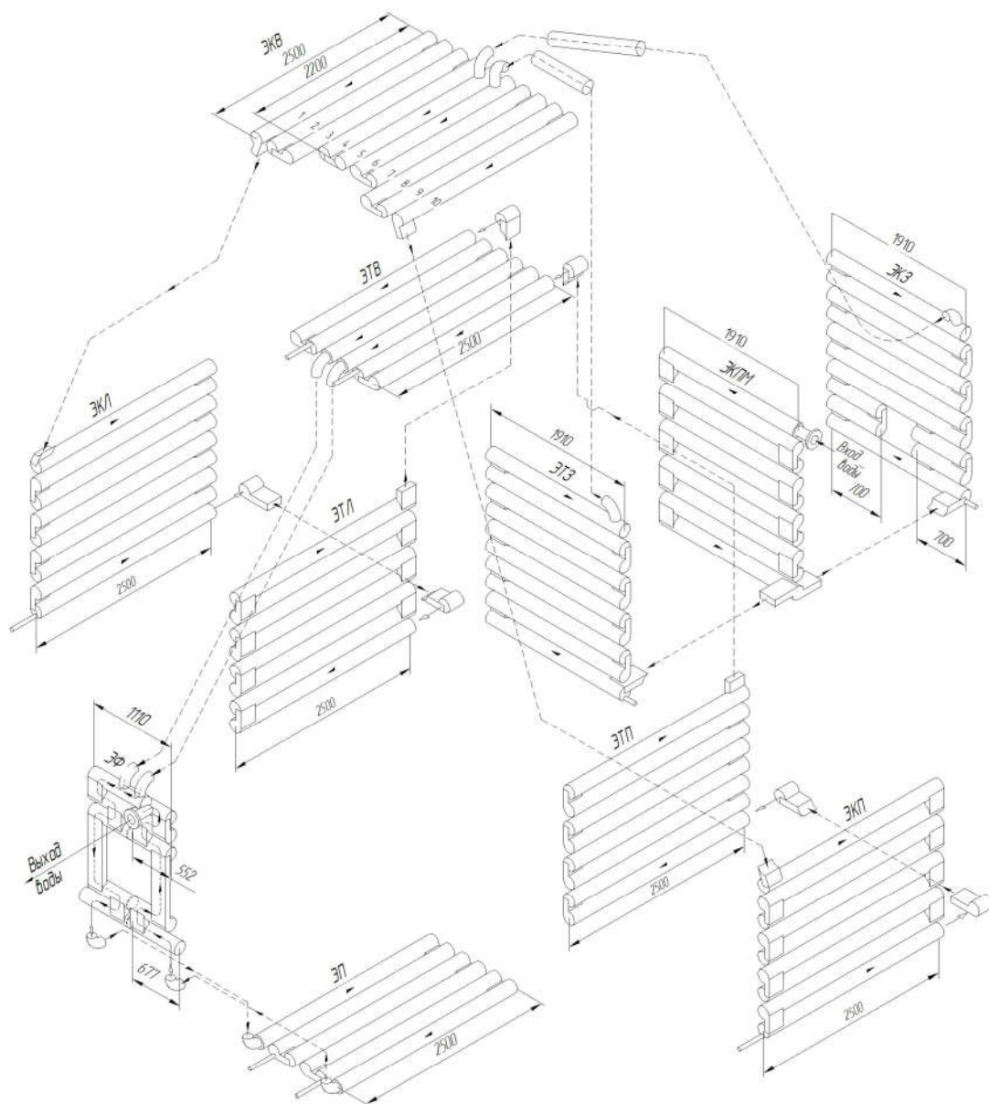
Схема гидравлическая КВа-1,74ГМ.
