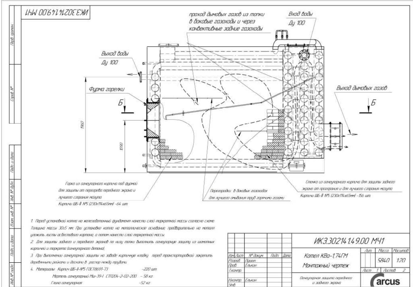
Рис.5 Монтажный чертёж КВа-1,74ГМ
