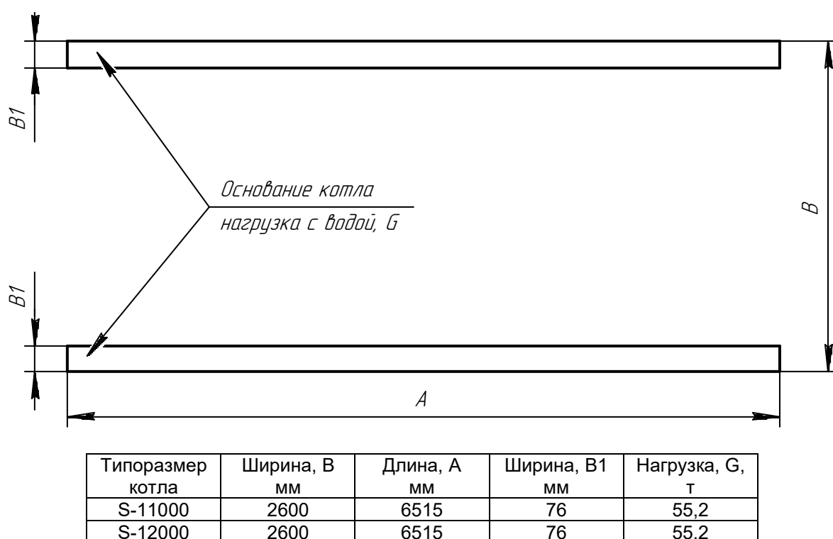
Рисунок 7. Фундамент котла.
