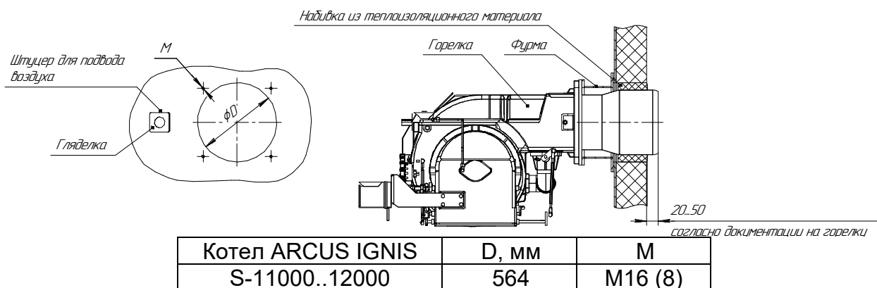
Рисунок 2. Отверстие под горелку
