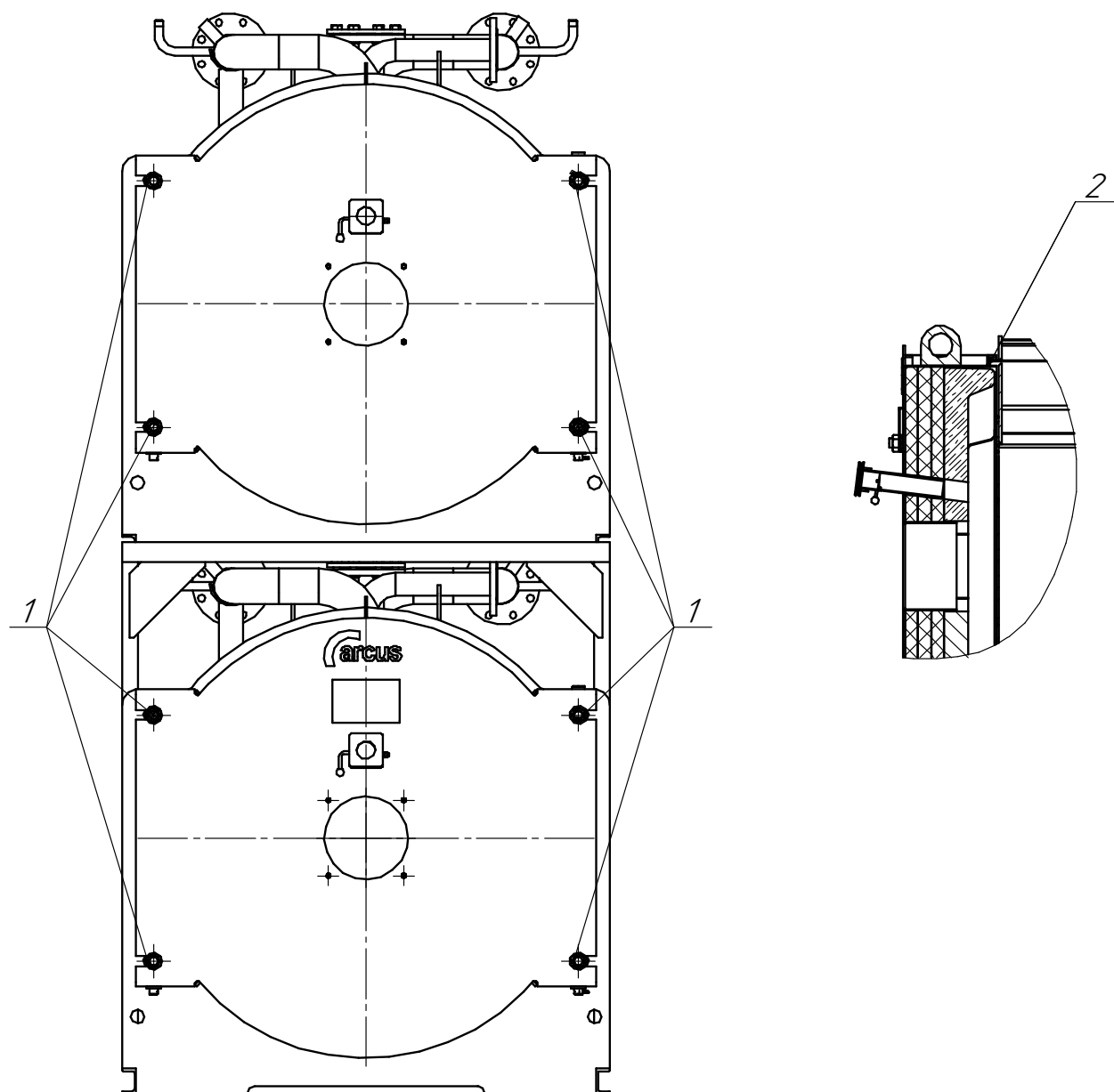
Рисунок 10. Передние крышки.
