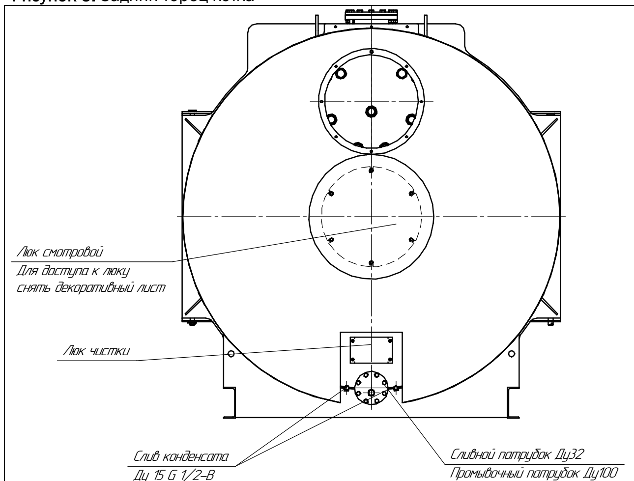
Рисунок 6. Задний торец котла
