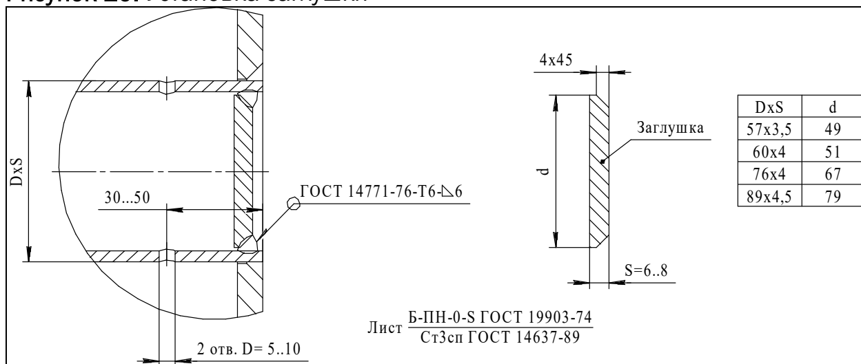
Рисунок 10. Установка заглушки
