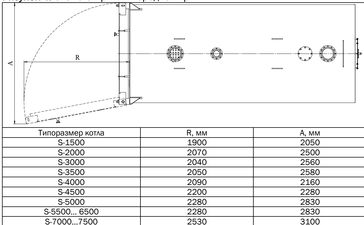
Рисунок 4. Схема открытия передней крышки
