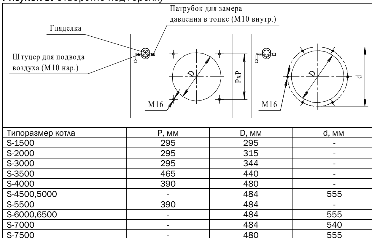
Рисунок 3. Отверстие под горелку
