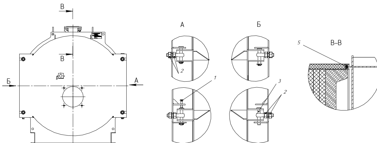
Рисунок 8. Передняя крышка.
