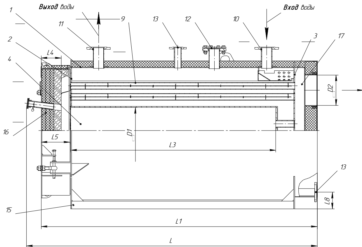
Рисунок 1. Схема котла
