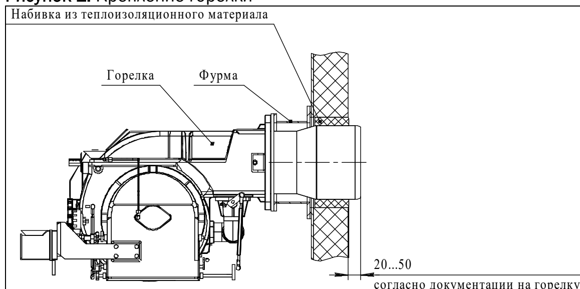
Рисунок 1. Крепление горелки
