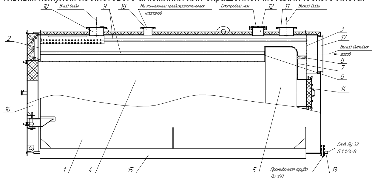
Рисунок 1. Схема котла
