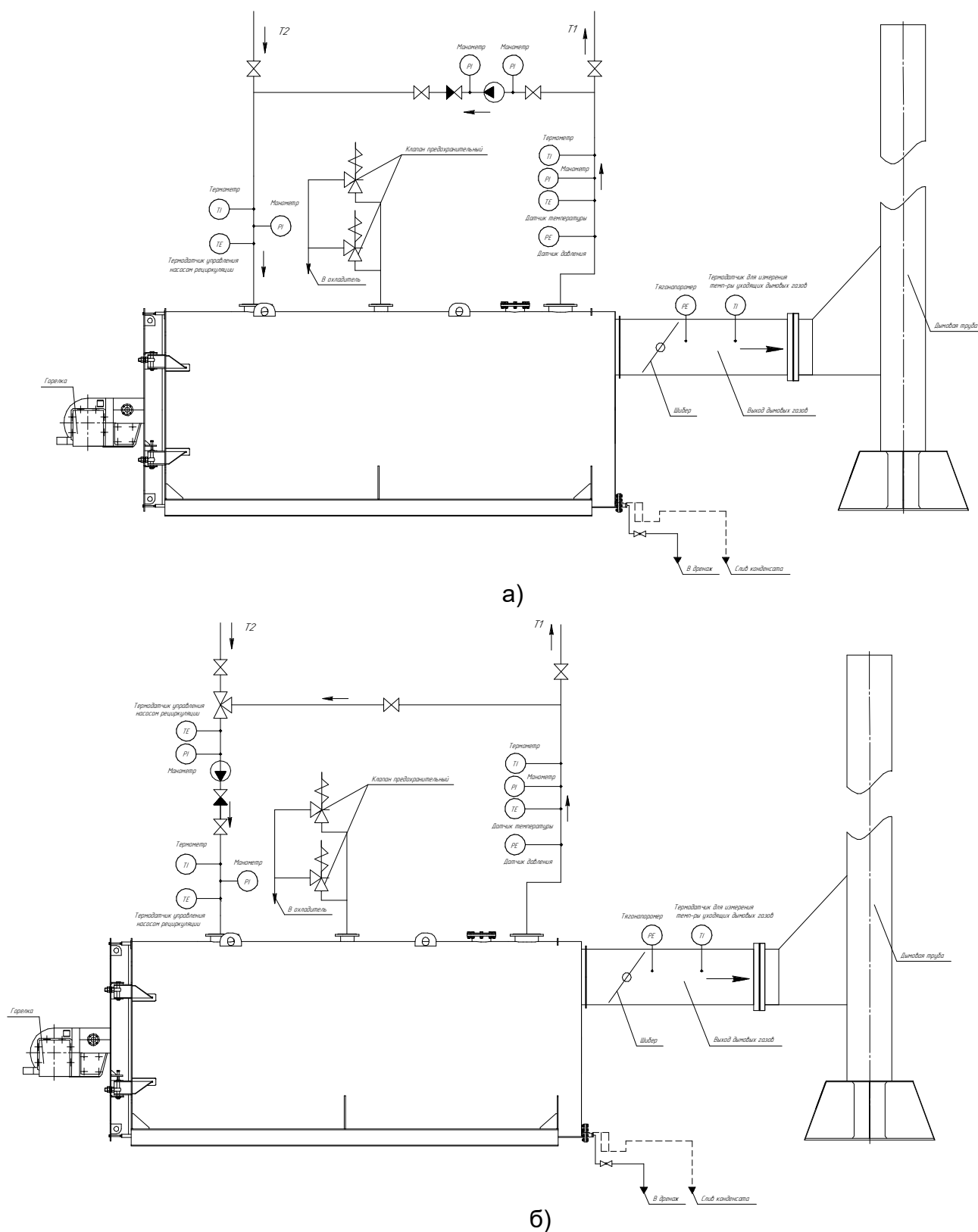
Рисунок 5. Принципиальные схемы включения котла а) с насосом рециркуляции; б) с трехходовым клапаном
