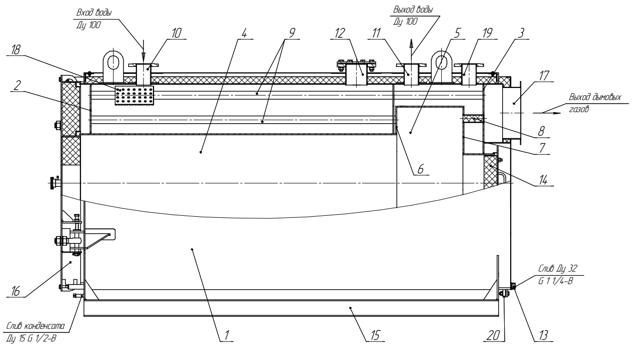
Рисунок 1. Схема котла
