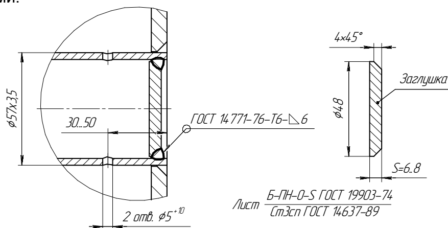
Рисунок 9. Установка заглушки.
