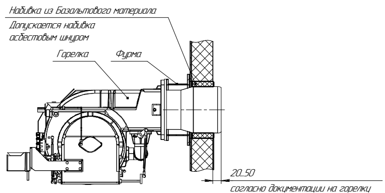
Рисунок 3. Крепление горелки
