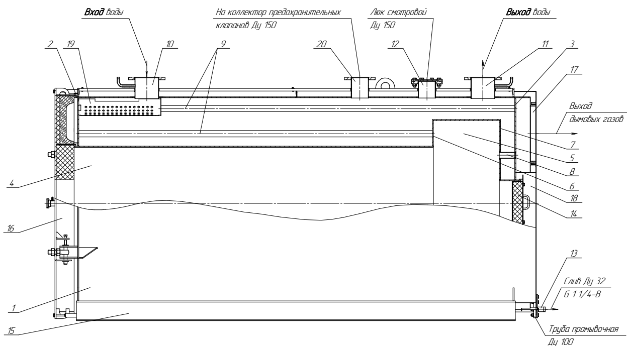
Рисунок 1. Схема котла
