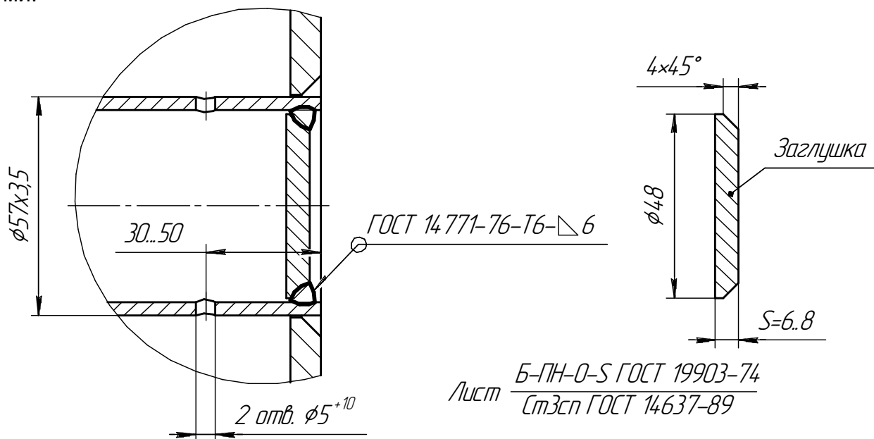
Рисунок 8. Установка заглушки.
