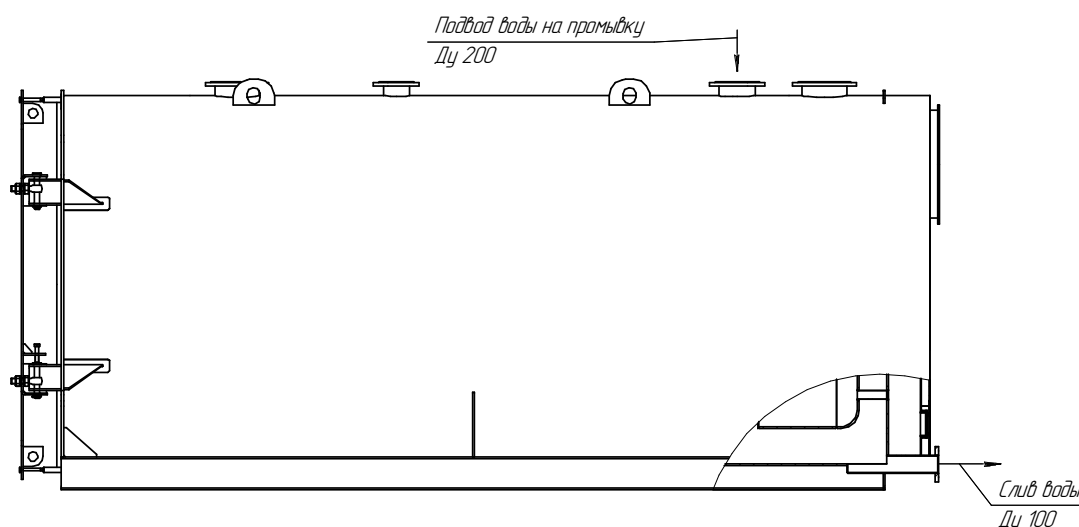
Рисунок 6. Вариант промывки котла.
