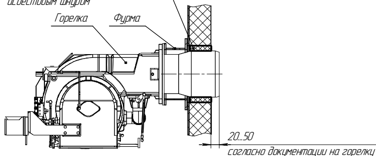
Рисунок 3. Крепление горелки
