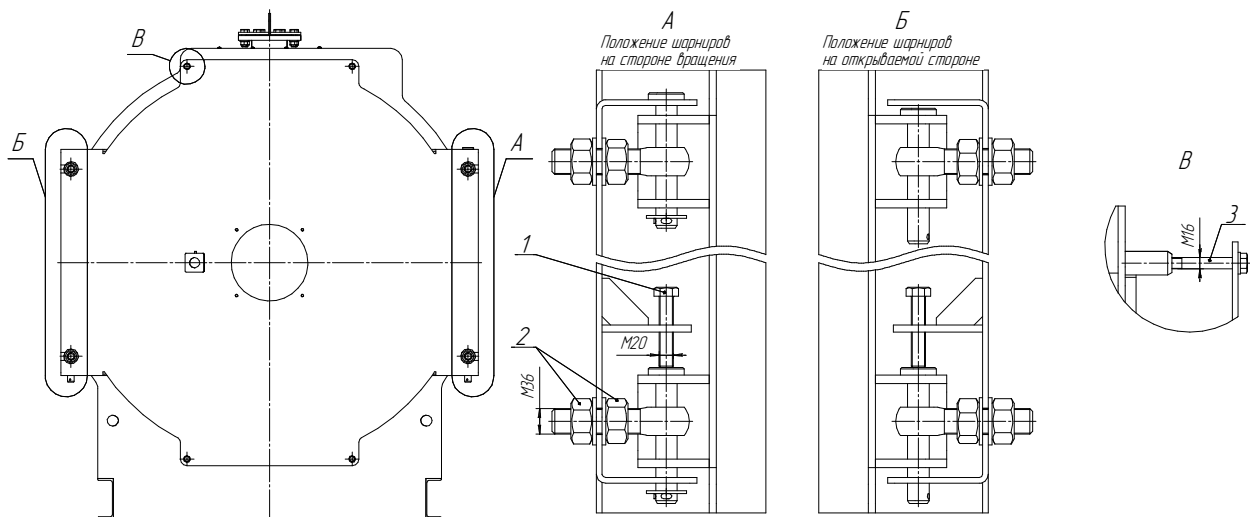
Рисунок 7. Передняя крышка.
