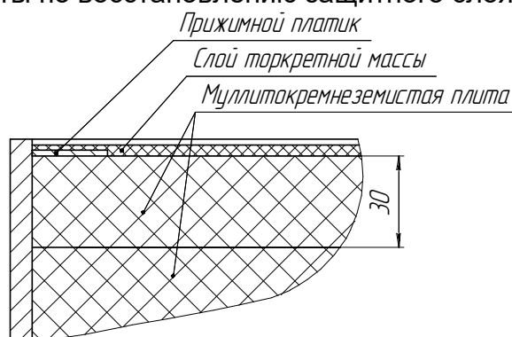
Рисунок 9. Разрез смотрового люка.
