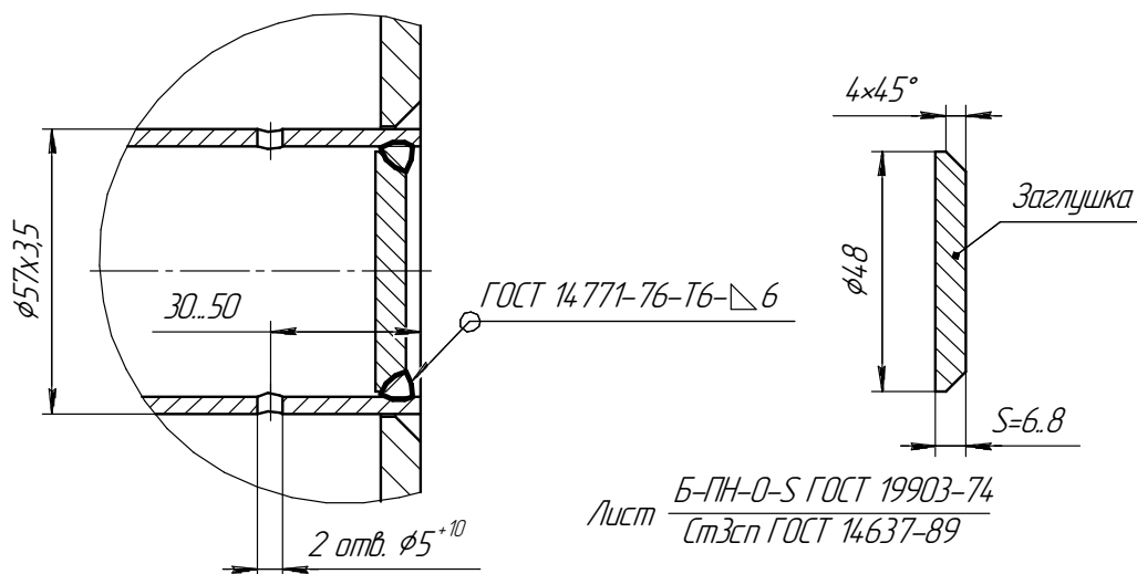
Рисунок 9. Установка заглушки. (Вариант для трубы 57х3,5)
