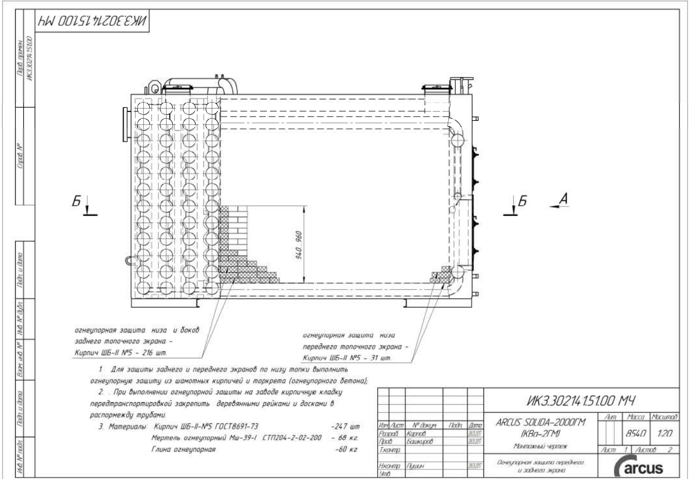
Рис.3 Монтажный чертёж
