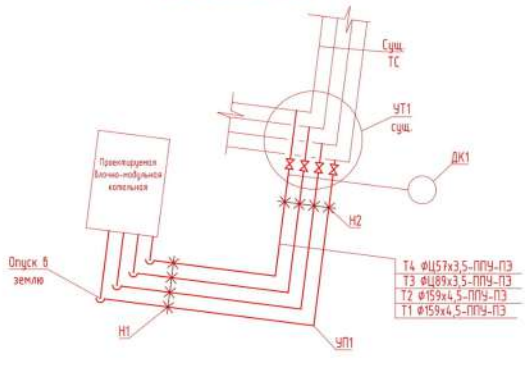
Схема тепловых сетей
