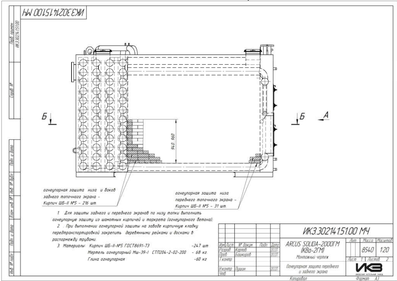
Рис.3 Монтажный чертёж
