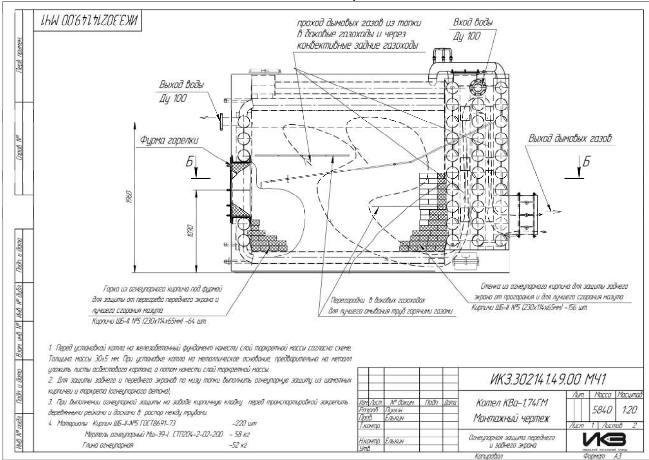
Рис.5 Монтажный чертеж КВа-1,74ГМ
