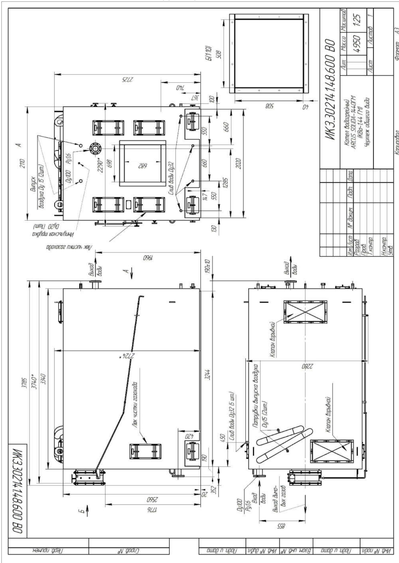
Рис.2 Вид общий котла КВа-1,44ГМ
