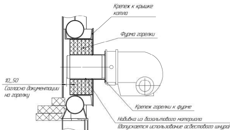
Рисунок 1. Крепление горелки.
