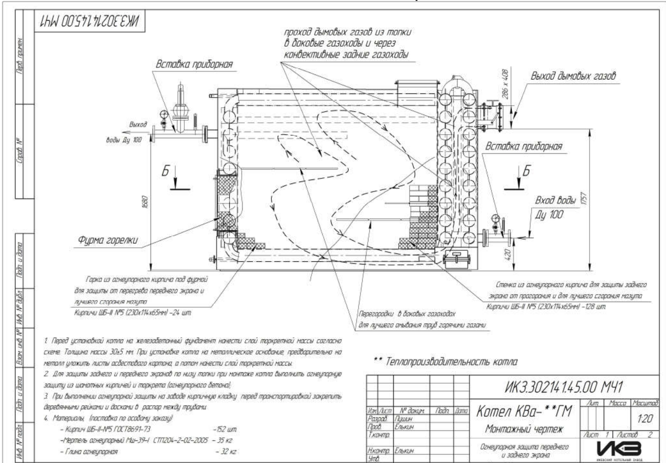
Рис.3 Монтажный чертёж
