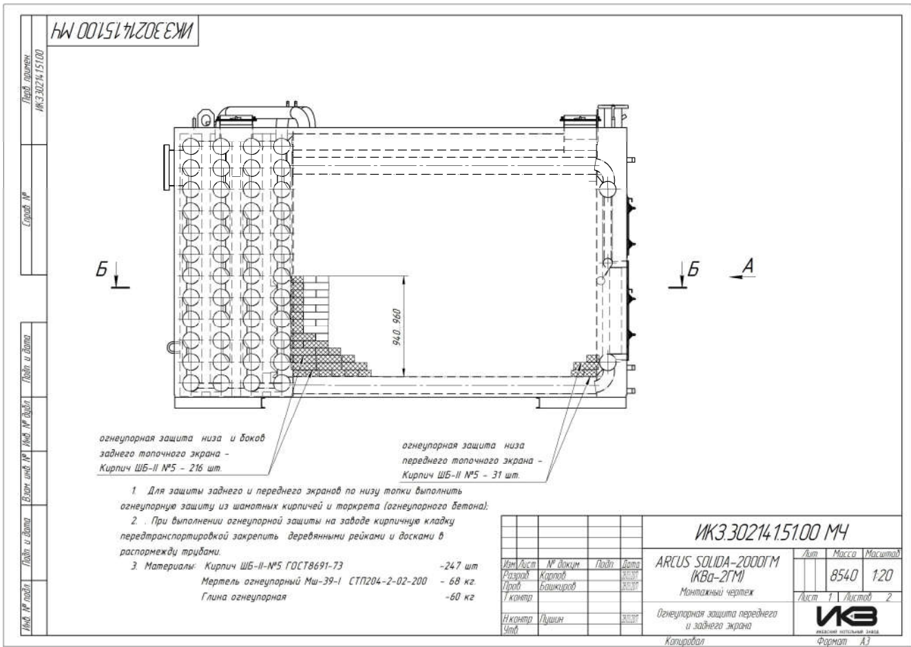
Рис.3 Монтажный чертеж
