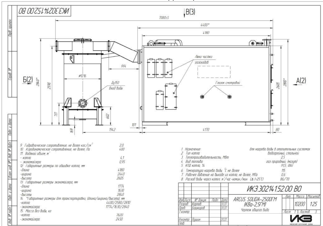
Рис.2 Вид общий
