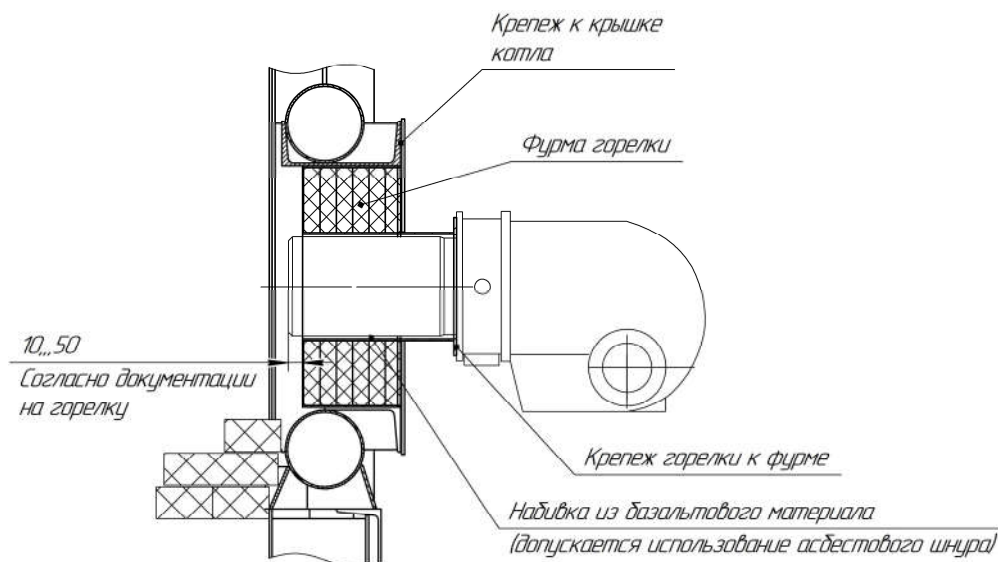
Рисунок 1. Крепление горелки.
