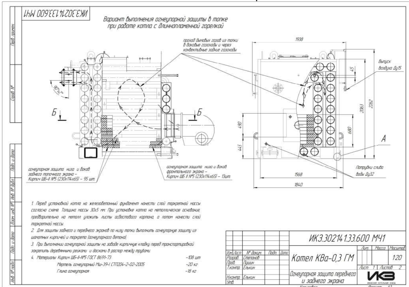
Рис.3 Монтажный чертёж
