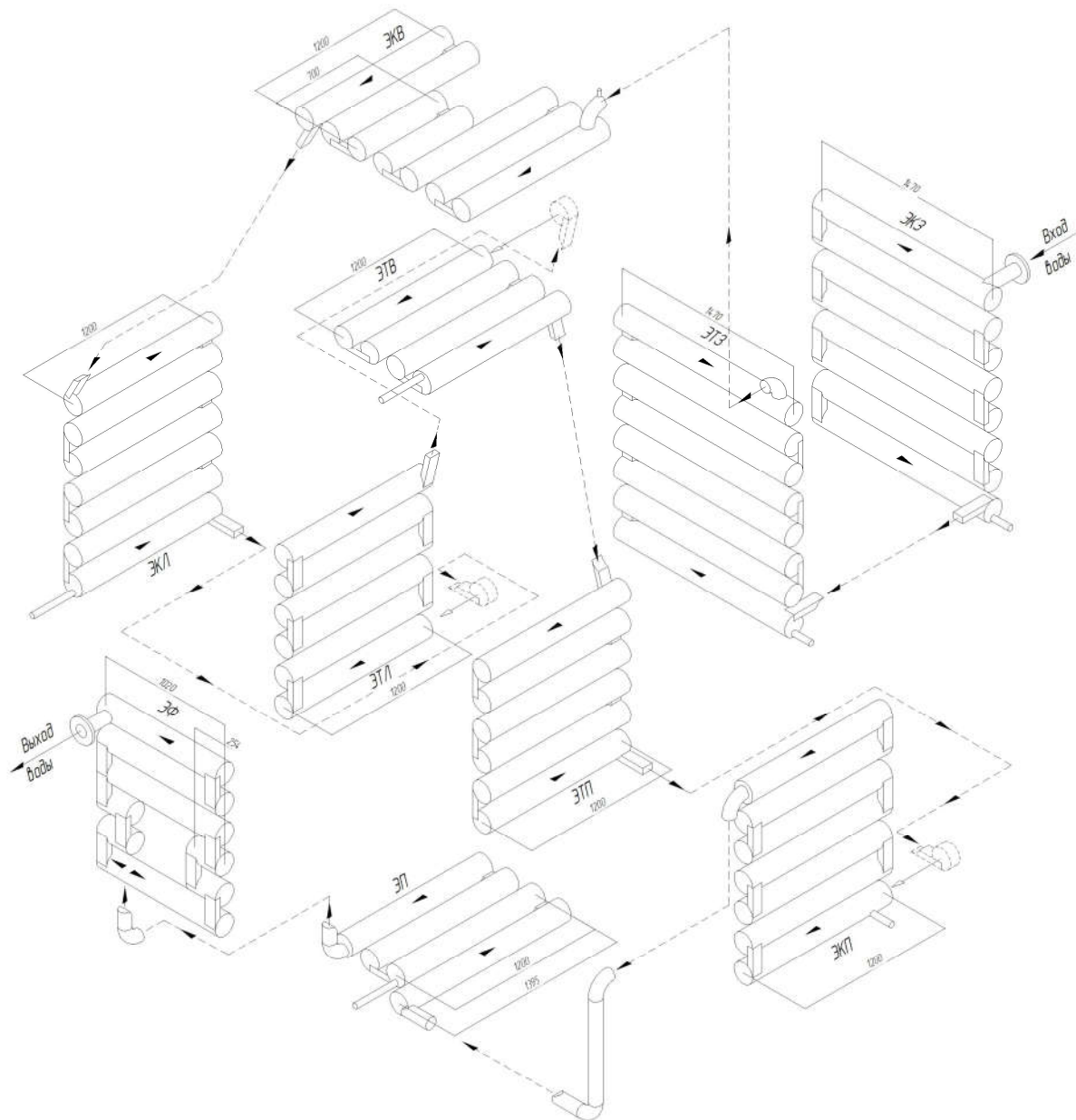
Схема гидравлическая КВа-0,3ГМ.
