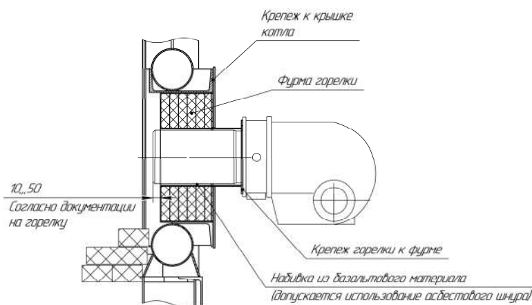
Рисунок 1. Крепление горелки.
